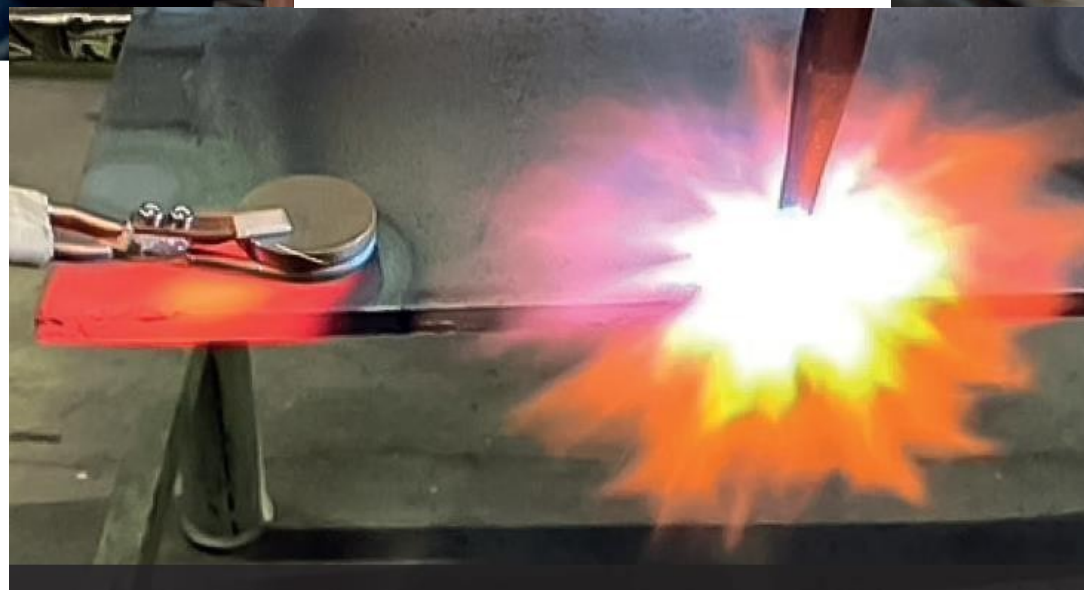
Srovnání ohřevu indukcí / kyslíkoacetylenem (autogen)
